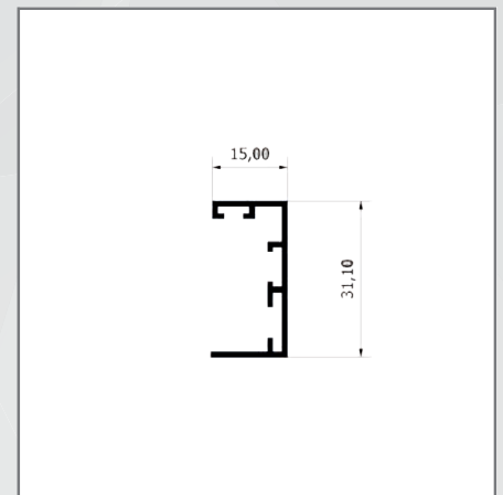
Profilo chiusura laterale
