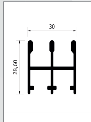
Telaio tre vie
