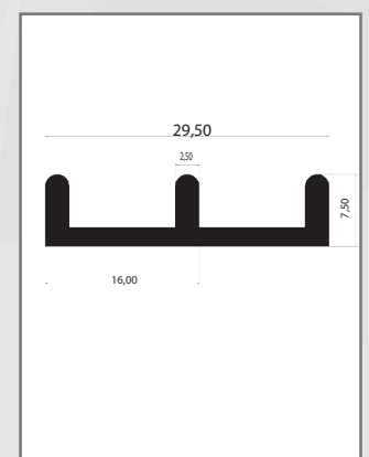
Guida bassa a tre binari
