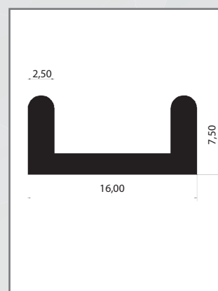
Guida bassa a due binari
