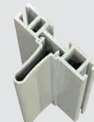
Profilo rinforzato maniglia laterale
