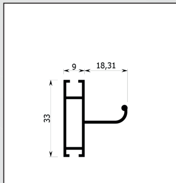
Maniglia saliscendi.
